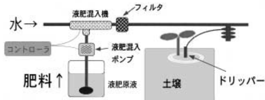
図1-4 Drip fertigation（養液土耕）の概念図 施肥量低減や根に負荷されるストレス軽減が期待される養液土耕法 液肥を適宜希釈し、植物の必要量に合わせて施用する。
