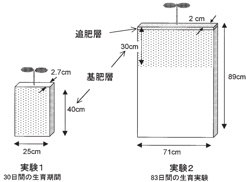
図3-1 実験に用いた根箱の外観図
