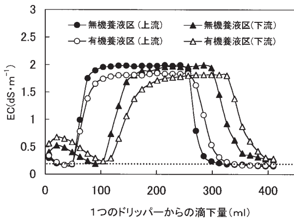
図4-10 液肥混入機の作動状態 設定としては、灌水量 1L \cdot h^{-1} であり、2分のプレリンスの後、11.4倍に希釈した無機液肥または、2.5倍に希釈した有機液肥を13分間導入した。その後、10分のリンスを行った。上流は最も水上のチューブ、下流は最も水下のチューブから滴下された液を示す。 図中の点線は水道水のEC ( 0.17dS \cdot m^{-1} )を示す。
