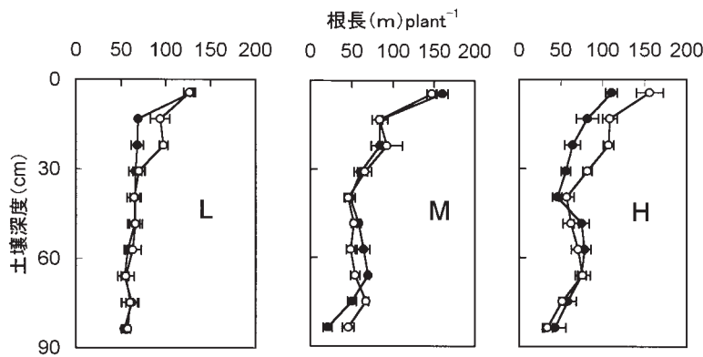
図3-8 肥料の種類および施肥濃度がトマトの根の垂直分布に与える影響
