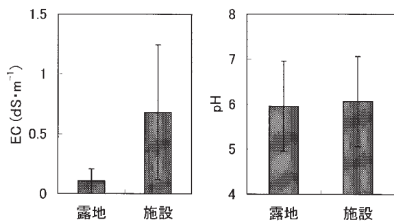
図 2-1 施設および露地土壌の EC と pH 表 2-1 の土壌について, 1:5 土壌抽出液の EC と pH を測定した。 露地 38 点, 施設 89 点の平均値を示す。縦棒は標準偏差。
