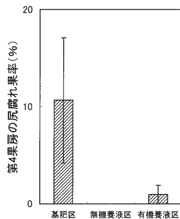
図 4-15 養液土耕法が尻腐れ果の発生率に及ぼす影響
