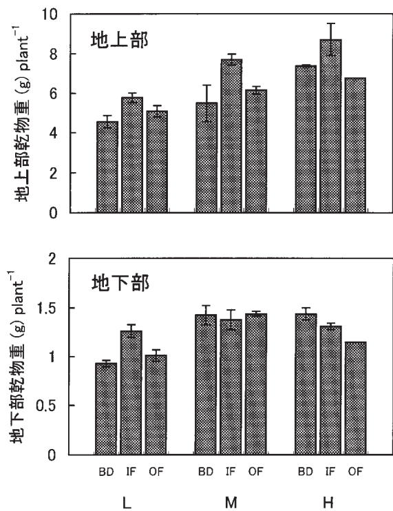
図4-2 養液土耕法によって栽培したトマトの地上部および地下部の乾物重
