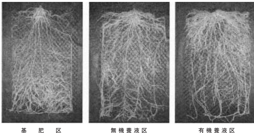
図4-4 養液土耕が根系形態に与える影響
