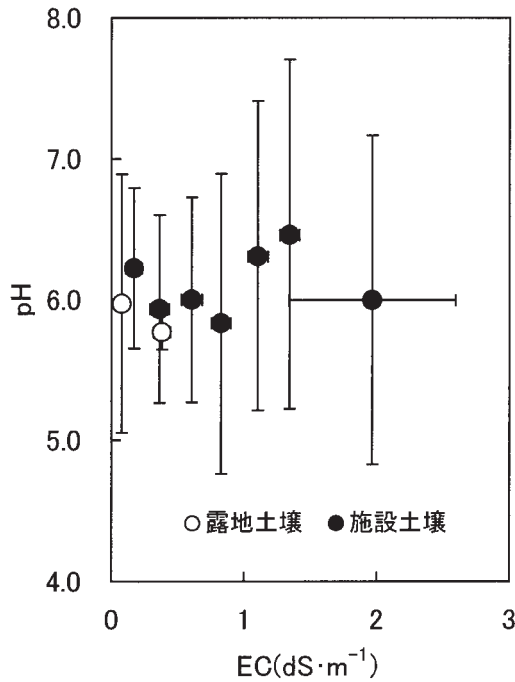
図2-2 露地および施設土壌におけるpHとECの関係
