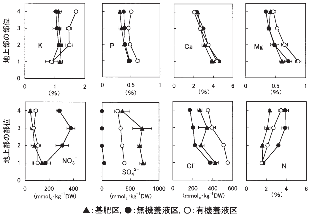
図4-17 トマト葉部の無機成分組成 3株の平均値, 横棒は標準誤差を示す.
