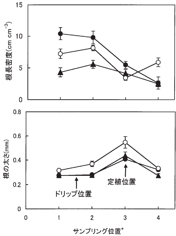
図4-20 養液土耕法が根の水平分布と太さに与える影響
