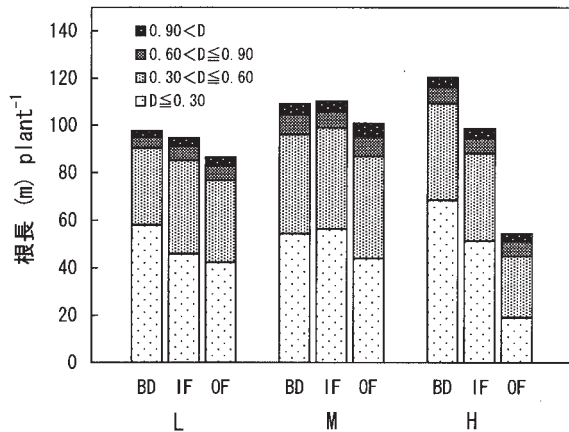
図4-3 養液土耕が大きさ別の根長に与える影響
