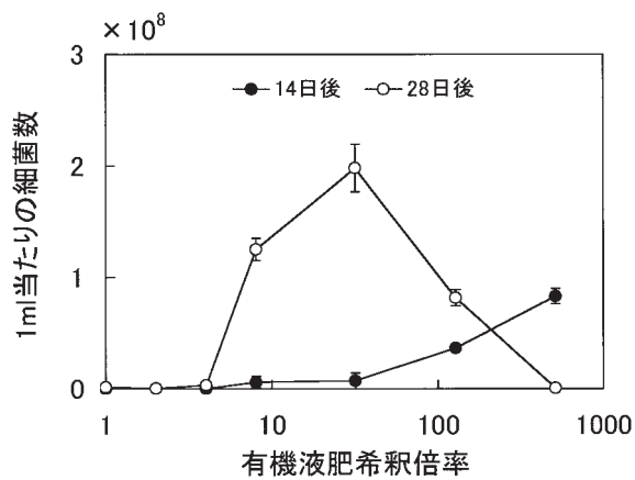
図4-9 有機液肥の希釈倍率および静置日数が細菌数に与える影響 縦棒は標準誤差を示す。(n=2)
