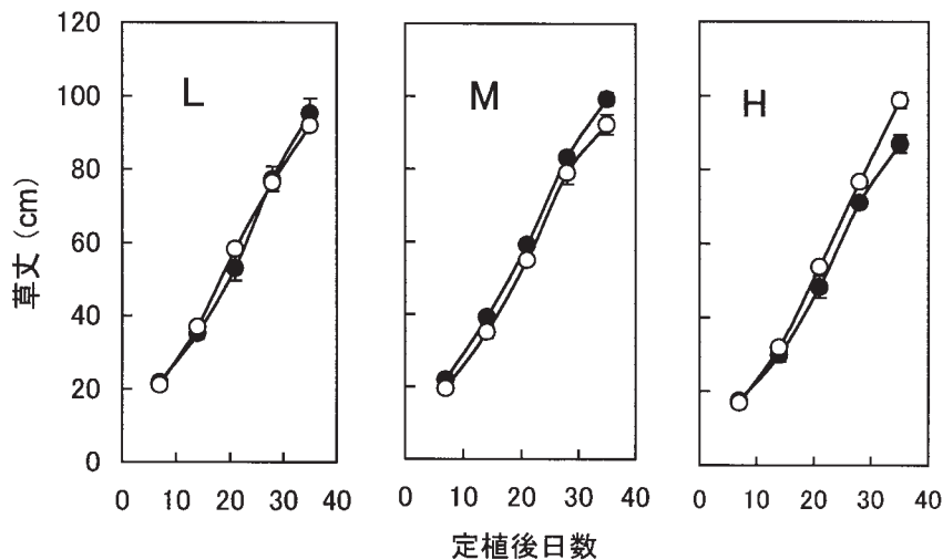
図3-5 肥料の種類および施肥濃度がトマトの草丈に与える影響
