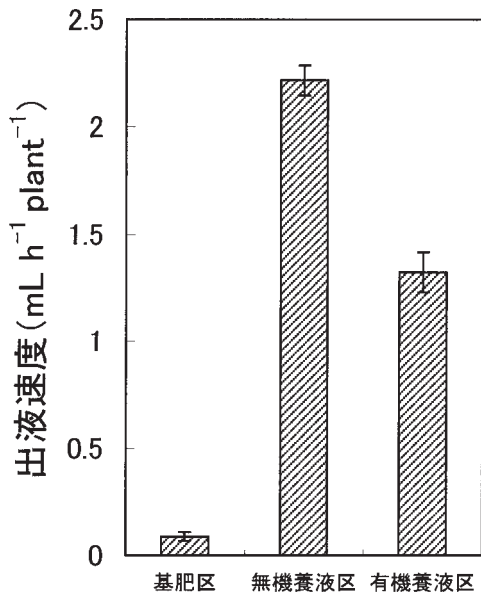
図4-18 栽培法が出液速度に及ぼす影響 出液速度の平均値 (n=8)。縦棒は標準誤差を示す。
