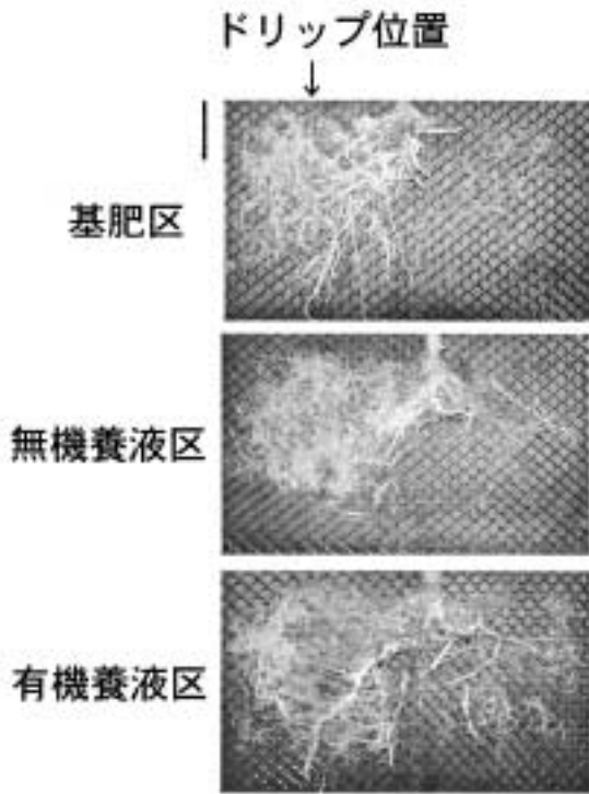
図4-19 養液土耕法が根系形態に与える影響 縦棒は5cm
