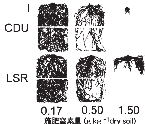
図 3-2 肥料の種類および施肥量がトマトの根系形態に与える影響
