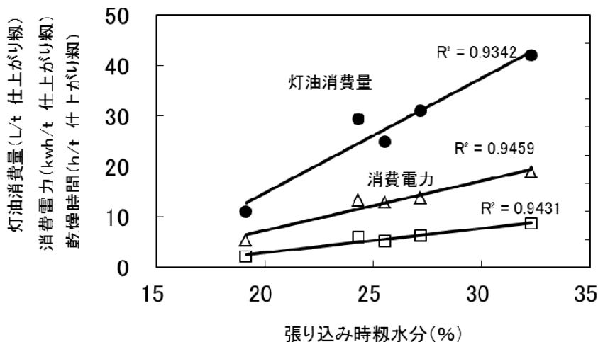
図2-14 張り込み時籾水分と灯油消費量、電力消費、乾燥時間の関係
