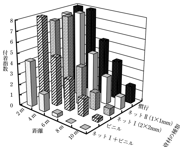
第1図 飛散防止資材と距離別薬剤付着量 (2003年)
