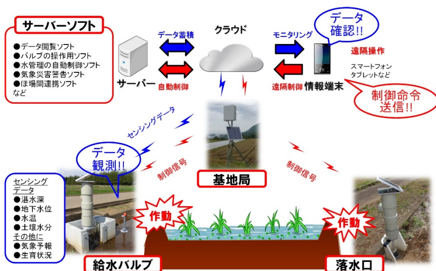
圃場水管理システムの概要
